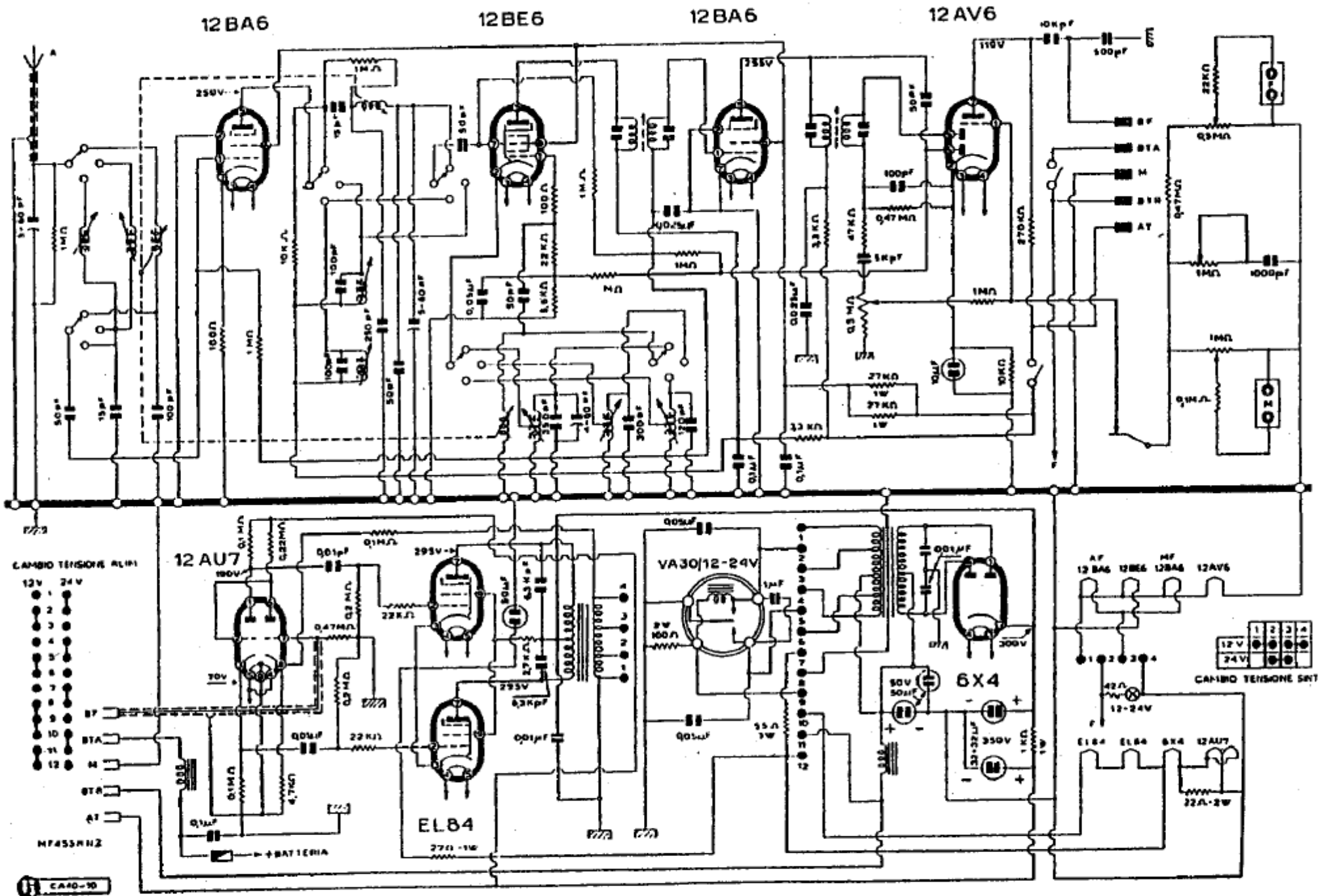
AUTOVOX - Autoradio Mod. RP 50
